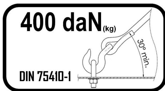
Rys. 2. Zasady obciążania uchwytów mocujących
